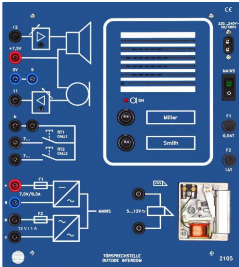
Türsprechstelle (Typ 2105)
